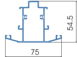
Đồ chia khung
