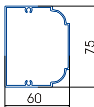
Nối đố 1154
