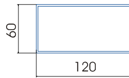
Khung bao cửa thủy lực 60x120
