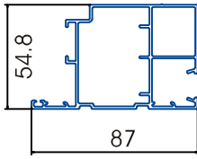
Cánh cửa đi xingfa liền sập mở ngoài
