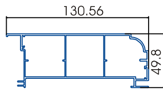
Nối khung bao xingfa liền phào
