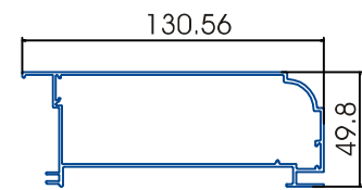
Nối khung bao xingfa liền phào
