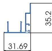
Móc cánh cửa lùa VP40HT
