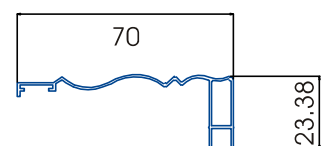
Óp phào cửa thủy lực 65
