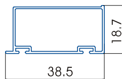
Ốp chân cánh cửa đi
