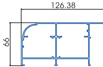
Nối khung bao xingfa liền phào 1001
