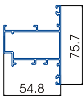
Thanh cánh cửa sổ xingfa không gân
