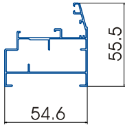
Khung bao cửa đi
