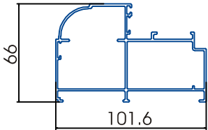
Khung bao xingfa liền phào 1001
