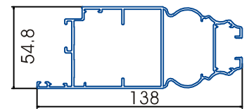
Cánh xingfa liền phào 140
