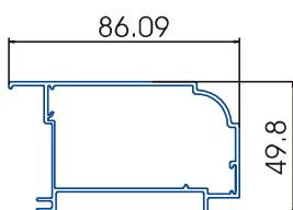
Nối khung bao xingfa liền phào tường 18
