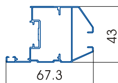
Cánh cửa sổ liền sập
