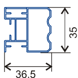
Trụ nhỏ
