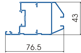
Cánh cửa sổ liền sập
