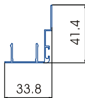
Móc cửa lùa Việt Ý
