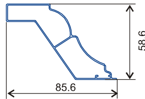
Phào nóc tủ
