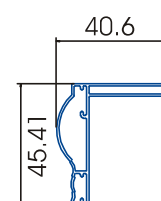
Phào bản
