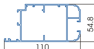
Cánh xingfa liền phào 110
