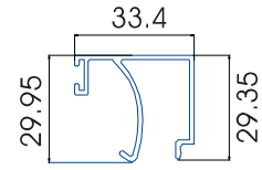
Sập cánh cửa thủy lực
