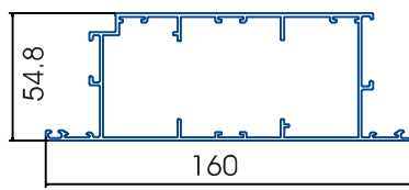
cánh xingfa bản 160 mở ngoài
