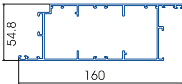
cánh xingfa bản 160 mở trong
