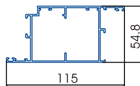
Cánh xingfa bản 120 mở trong
