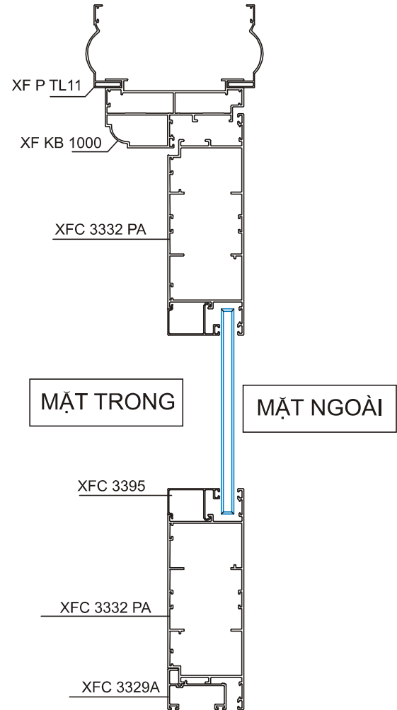
Mặt cắt 2 - 2
